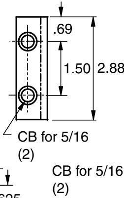
EF-30B
